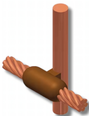
Conexión CR-3
